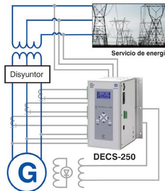
Figura 1: Diagrama de conexión para una aplicación típica del DECS-250
